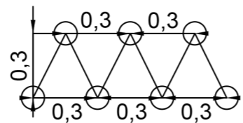
Схема посадки кизильника блестящего в двухрядную живую изгородь
